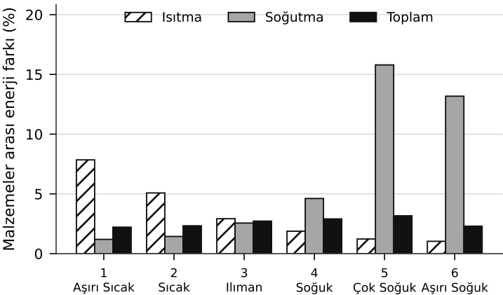
Şekil 5. Isıl kütlenin enerji ihtiyacına etkisi
